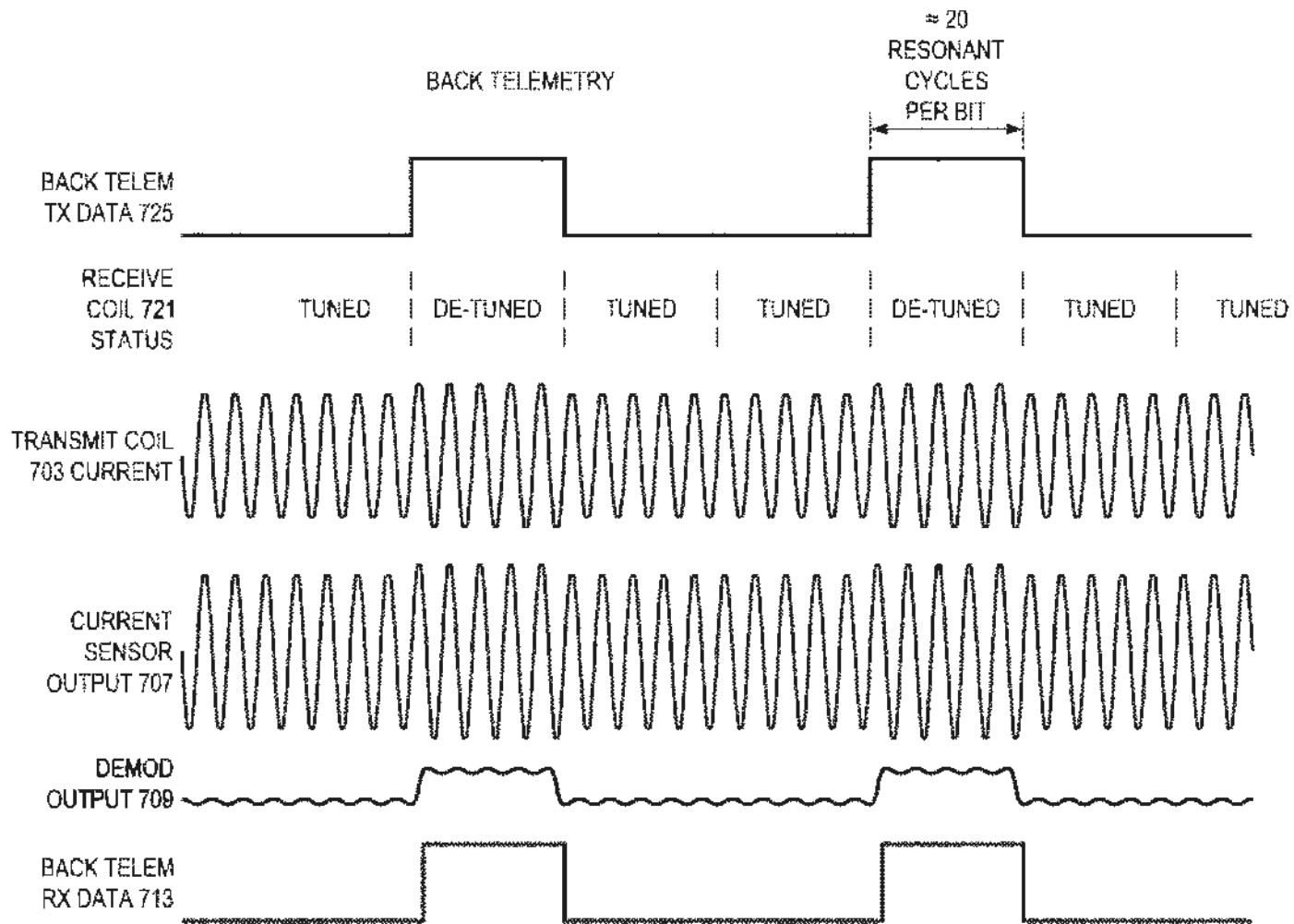
FIG. 14B
