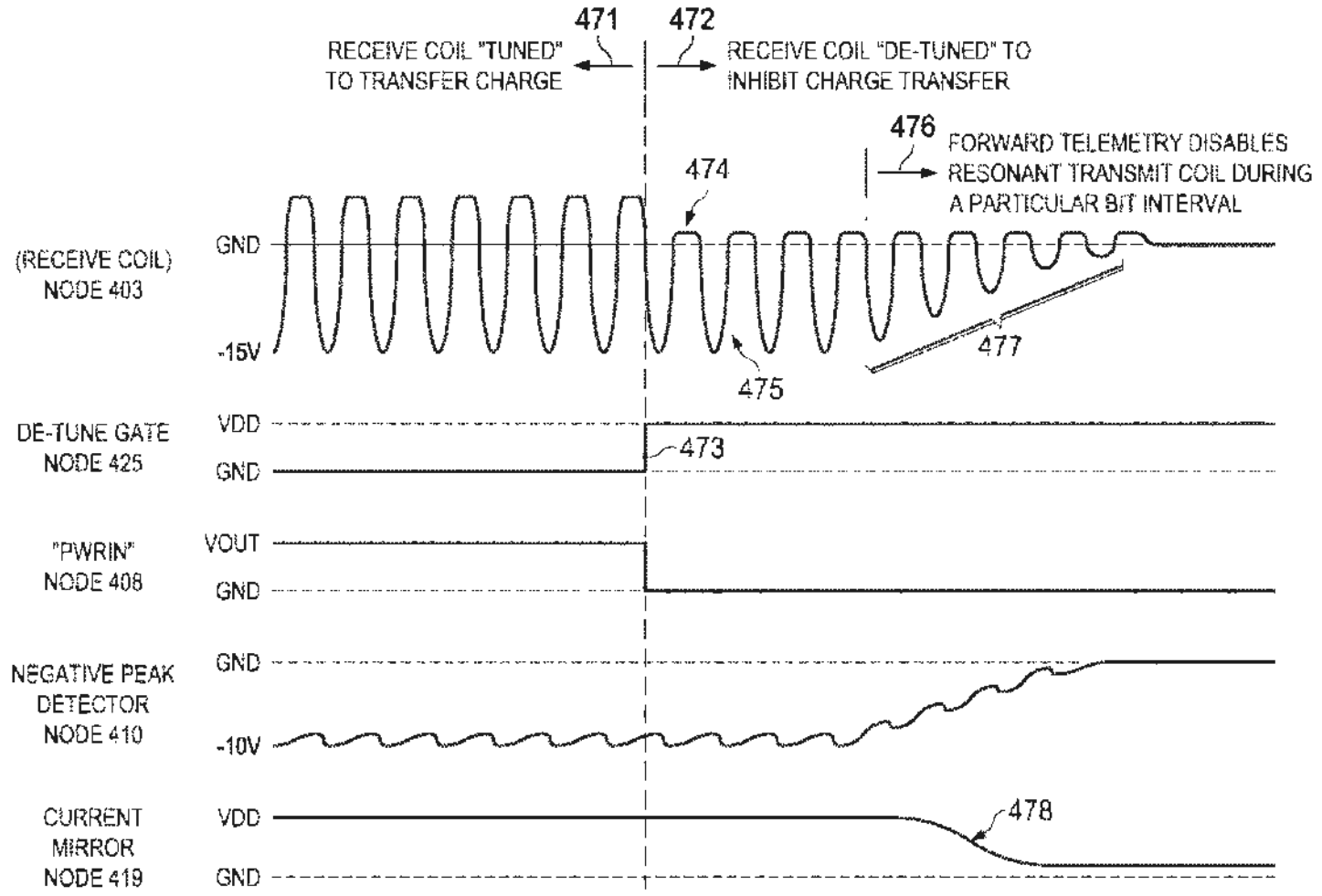
FIG. 23B
