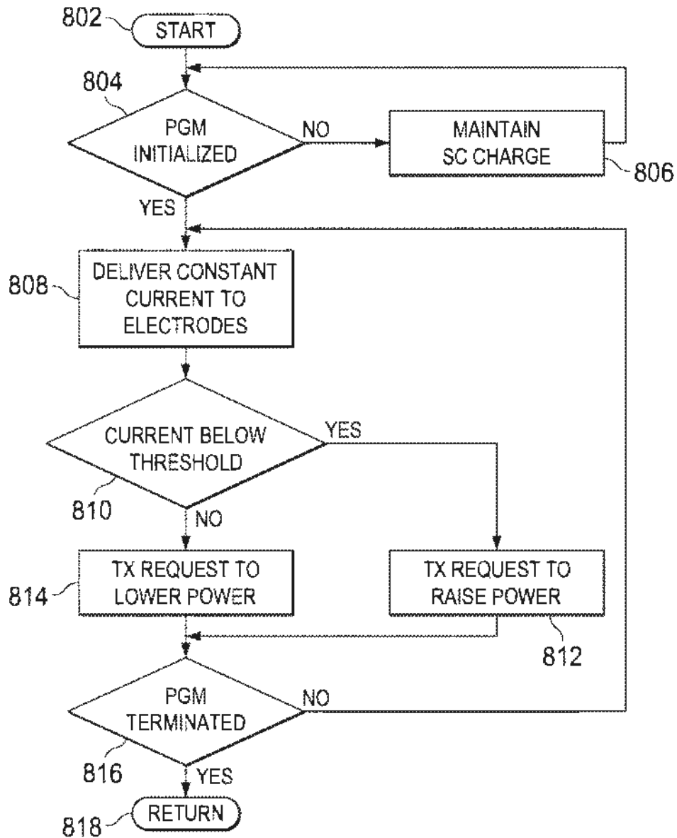
FIG. 22B
