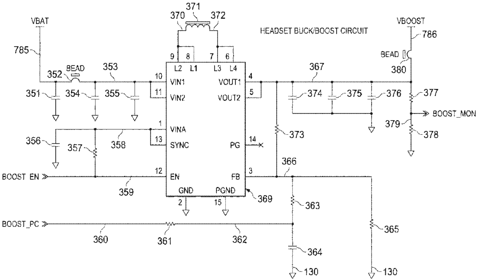
FIG. 20
