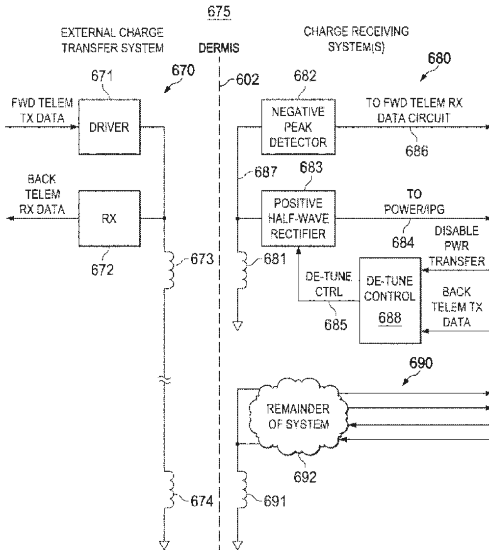
FIG. 13A
