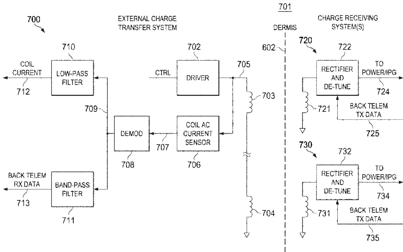
FIG. 14A
