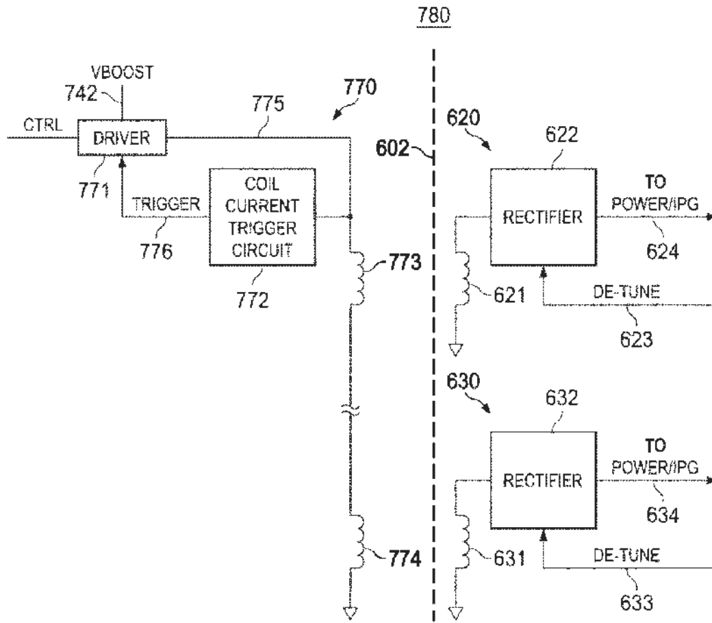
FIG. 16A
